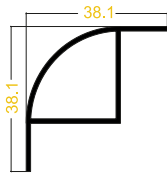
CUARTO DE CIRCULO 2 ALETAS REF: T-281
