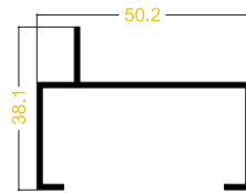
CANAL DE 2x1" ALETA SUPERDESCENTRADA REF: U-089
