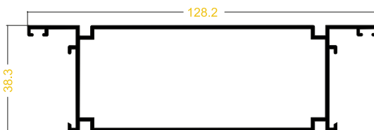
TUBULAR DE 3x1 1/2" CON DOBLE ADAPTADOR REF: 1104
