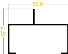
CANAL DE 2x1" ALETA DESCENTRADA REF: U-066
